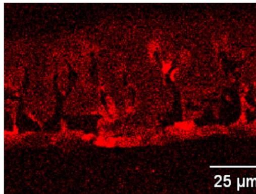
Verteilung Silber
