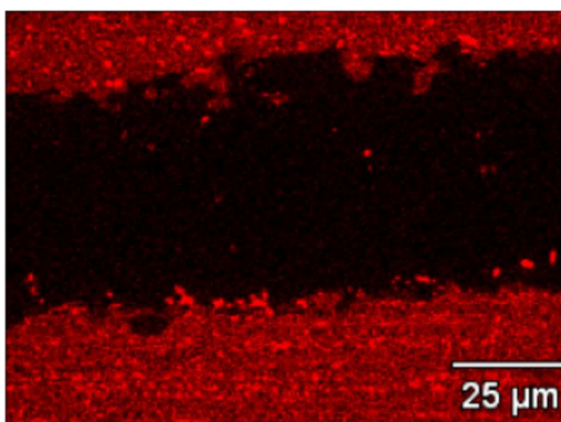
Verteilung Eisen
