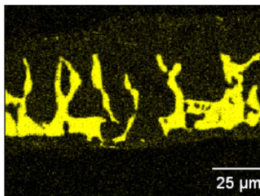
Verteilung Phosphor
