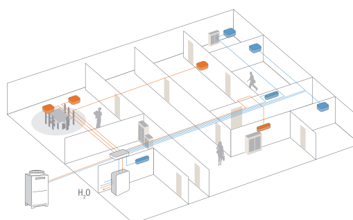
Das Funktionsprinzip des wirtschaftlichen 2-Leitersystems mit Wärmerückgewinnung zum gleichzeitigen Kühlen und Heizen.
