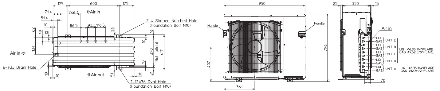
MXZ-5F102VF
