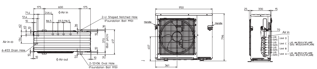
MXZ-4F83VF
