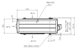
MUZ-Inverter Außengeräte, Kühlen/Heizen, MUZ-LN50VG2
