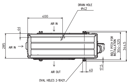
Außengeräte Standard Inverter SUZ-M60/71VA
