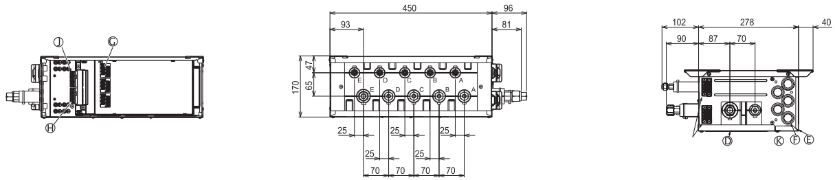
PAC-MK53BC
