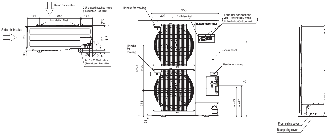
Außengeräte neue Generation Zubadan Inverter PUHZ-SHW112 / 140VHA-A / YHA-A
