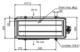
MUZ-Inverter Außengeräte, Kühlen/Heizen, MUZ-AP20-42VG
