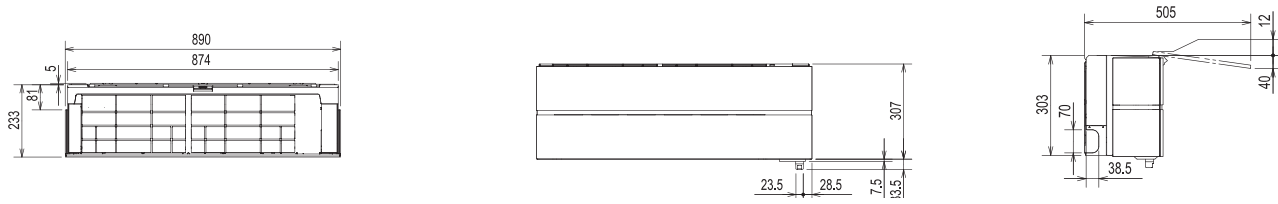
MSZ-Inverter-Wandgeräte Diamond, Kühlen/Heizen, MSZ-LN18-60VG2 R/V/W/B
