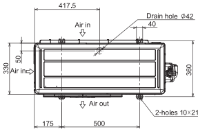
MUZ-Inverter Außengeräte, Kühlen/Heizen, MUZ-LN50VGHZ / 60VG
