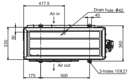
MUZ-Inverter Außengeräte, Kühlen/Heizen, MUZ-AP50VG
