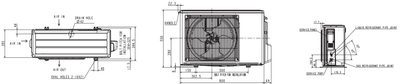
Außengeräte Standard Inverter SUZ-M35VA
