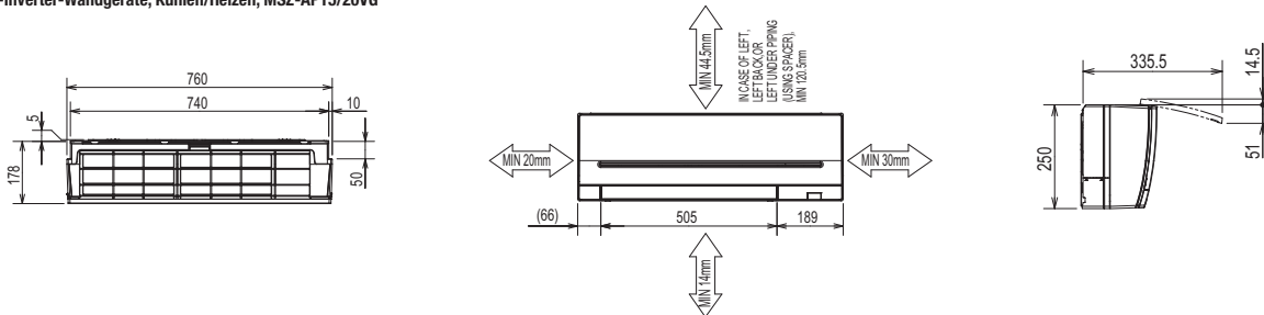
MSZ-Inverter-Wandgeräte, Kühlen/Heizen, MSZ-AP15/20VG
