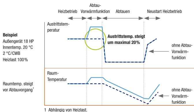
Abtau-Vorwärmfunktion ON/OFF
