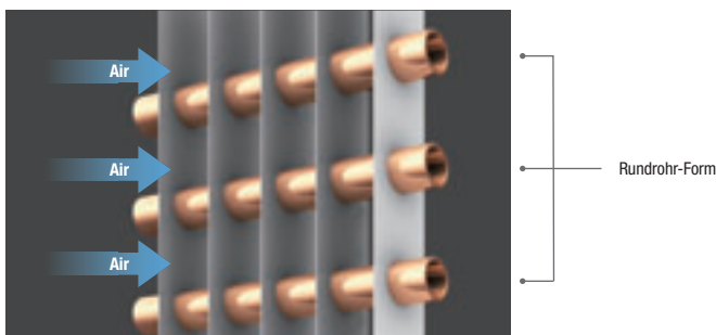
Rundrohr-Wärmetauscher
