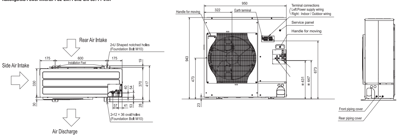
Außengeräte Power Inverter PUZ-ZM / PUHZ-ZRP60 / 71 VHA
