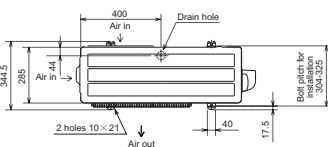
MUZ-Inverter Außengeräte, Kühlen/Heizen, MUZ-EF25 – 42VG
