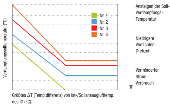
Energieeffiziente Verdampfungskontrolle
