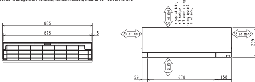
MSZ-Inverter-Wandgeräte Premium, Kühlen/Heizen, MSZ-EF18-50VGK W/B/S
