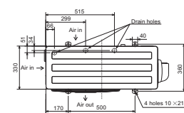
MUZ-Inverter Außengeräte, Kühlen/Heizen, MUZ-EF50VG
