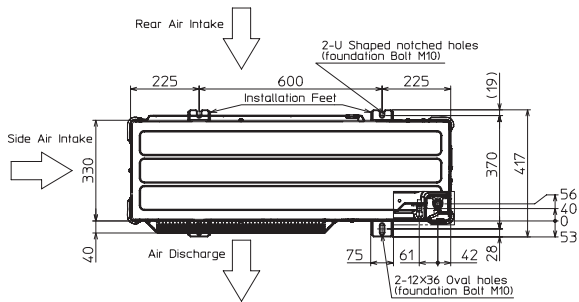
Außengeräte Power Inverter PUZ-M200/250YKA
