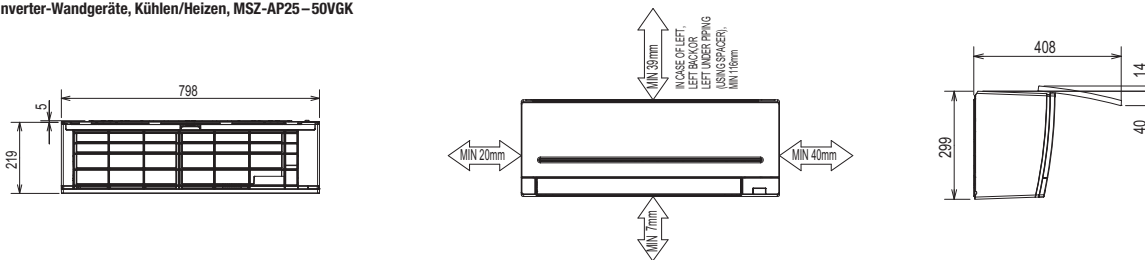
MSZ-Inverter-Wandgeräte, Kühlen/Heizen, MSZ-AP25-50VGK
