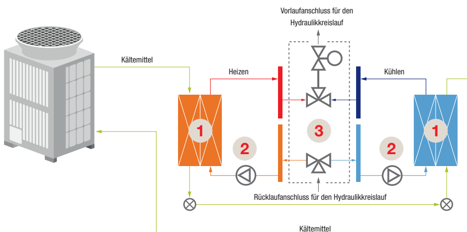
HBC-Übersicht
