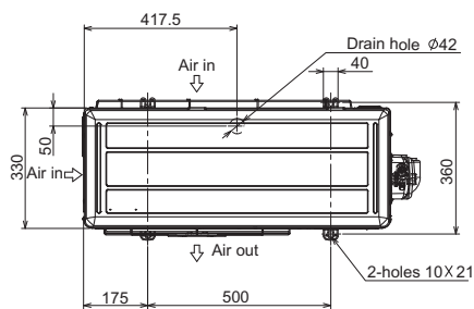
Außengeräte Standard Inverter PUZ-M100-140VKA/YKA
