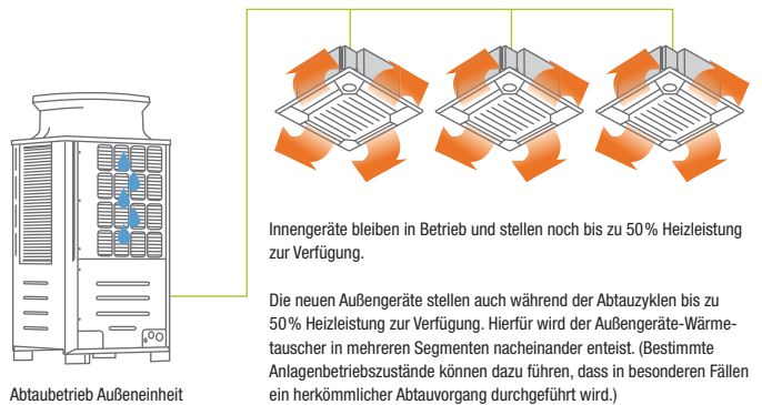
Abtaubetrieb Außeneinheit
