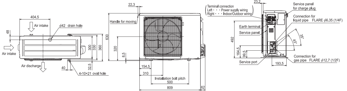
Außengeräte Power Inverter PUZ-ZM35 / 50 VKA
