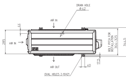
MUZ-Inverter Außengeräte, Kühlen/Heizen, MUZ-LN25 / 35VG2 / VGHZ2
