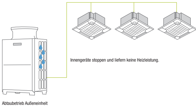
Abtaubetrieb Außeneinheit
