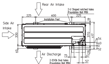
Außengeräte Standard Inverter PUZ-M100-140VKA/YKA
