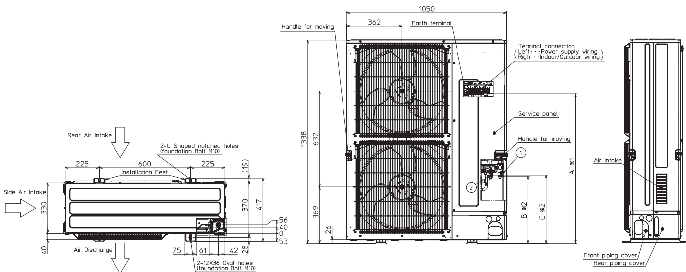
Außengeräte Power Inverter PUZ-ZM / PUHZ-ZRP100 – 140 YKA
