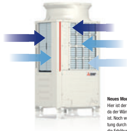
Herkömmliches Modell (YLM) In Bereichen, die weiter vom Lüfter entfernt sind, wird der Luftdurchsatz wegen des dreiseitigen Luftansaugsystems und des vertikal positionierten langen Wärmetauschers vermindert.
