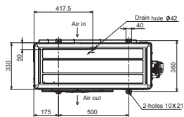
MUZ-Inverter Außengeräte, Kühlen/Heizen, MUZ-AP60/71VG
