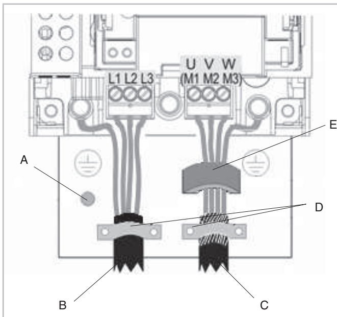
Abb. 10: Leistungsanschlüsse (Stromkabel und Motorkabel) mit Halterung
