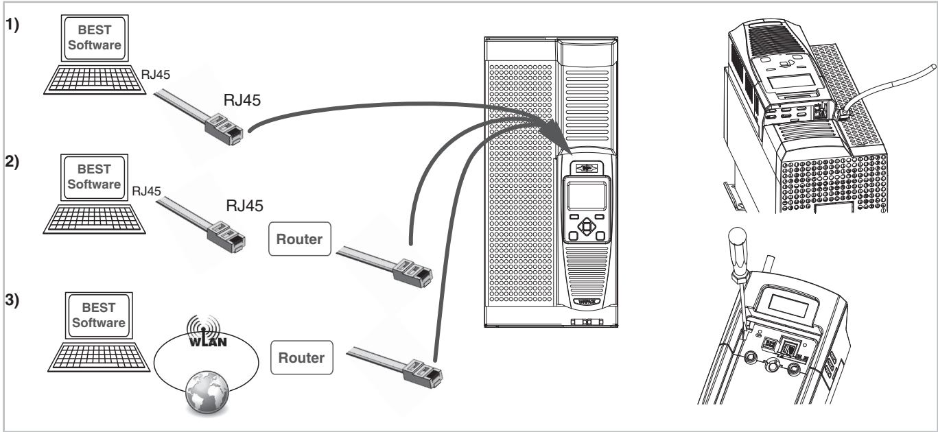
Abb. 19: Netzwerkkabel in den RJ45 Anschluss am VARIPACK einstecken und trennen
