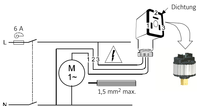
Abbildung 4: Anschluss
