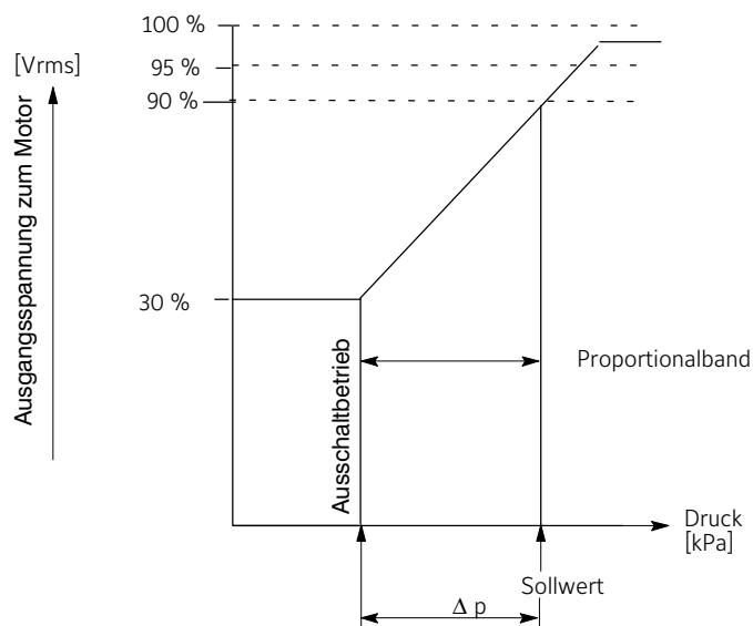
Abbildung 8: Regelcharakteristik der Drehzahlregler P215PR, P215RM
